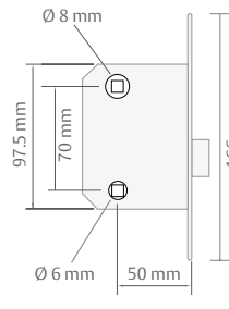
Picaporte Unificado Baño
